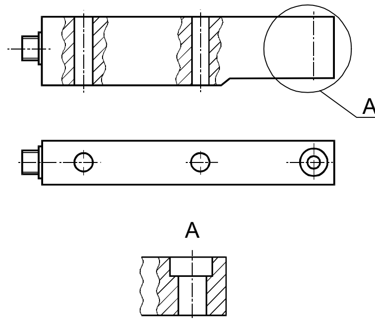
Рисунок Б.3 – Датчик силоизмерительный тензорезисторный консольный сдвиговый 4184 ДСТ
